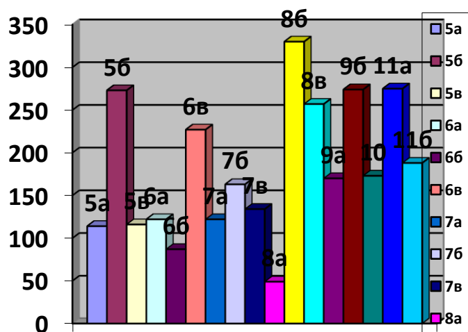
Диаграмма по результатам рейтинга участия классов в спортивных мероприятиях на уровне основного общего образования
